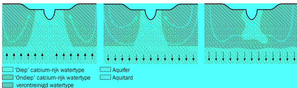
Figuur 6.5 Diepe kwel wordt als gevolg van de daling van de diepe stijghoogte vervangen door lokale kwel (Stuurman, 2000).
